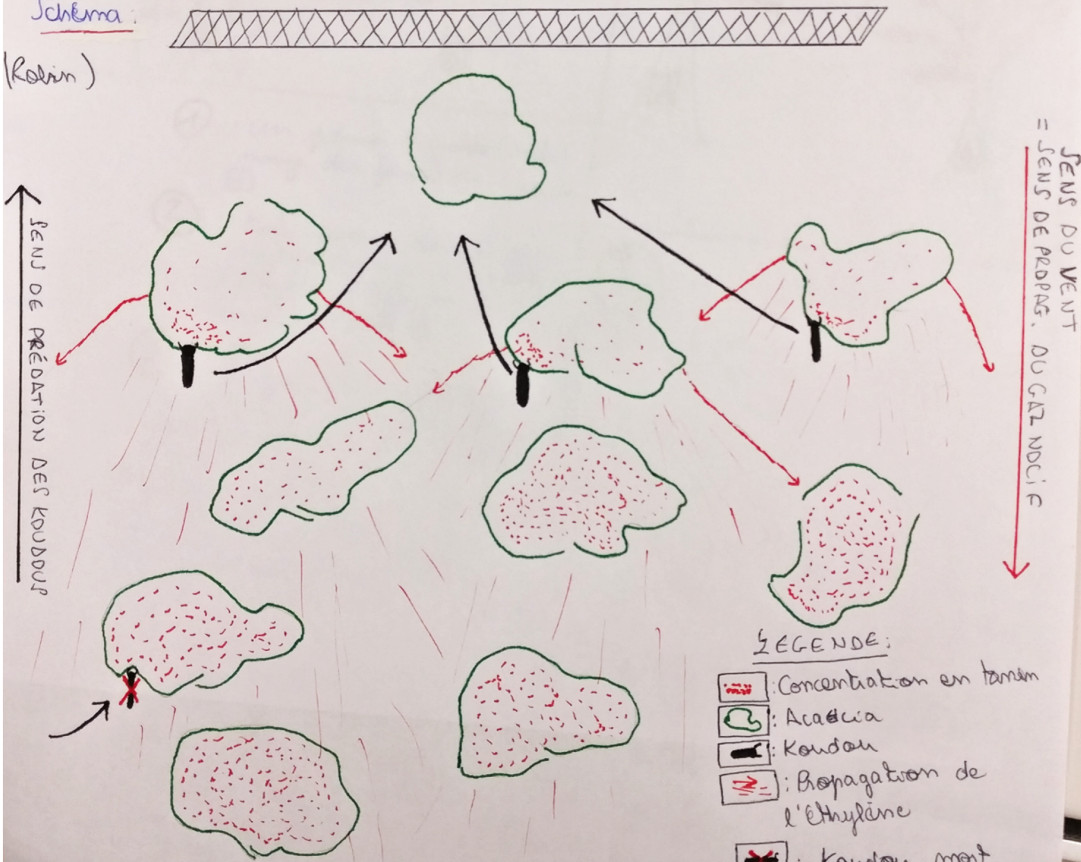
Schema de la strategie des acacias pour resister aux herbivores, appliquee dans un savan
